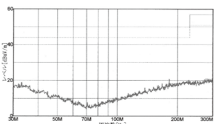
〈サンフレキ ROBO Type NSBS〉
