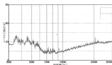
〈ケーブルのみ〉
